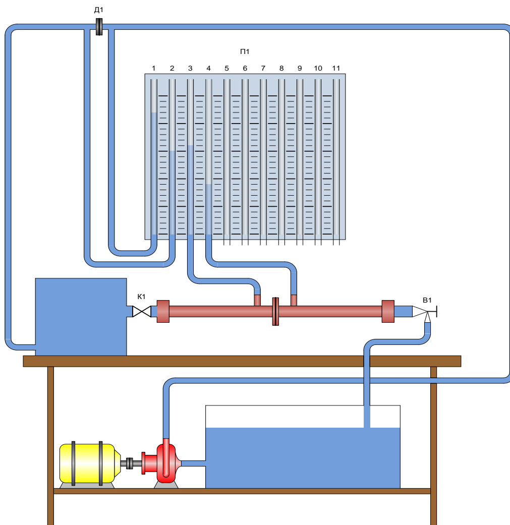
Рис. 1. Схема лабораторного стенда
