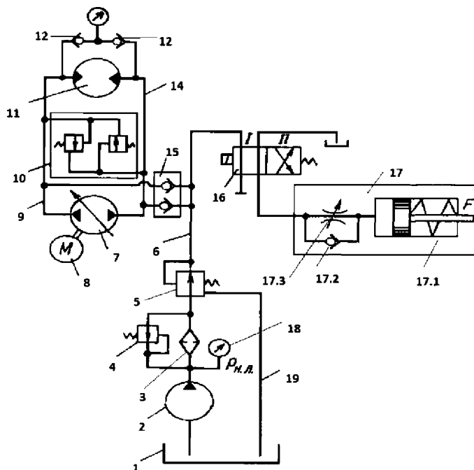
Рис. 1. Схема гидропривода лебедки крана
